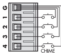
9) Branchement poussoir gong
