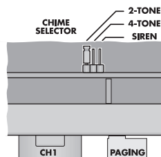
⑩ Wahl des Gongklanges
