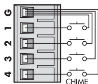
⑨ Anschluss Gongtaster
