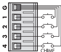
9 Conexión del pulsador chime
